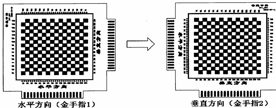
图 7 液晶板方向 (视角为正视液晶屏凸起面)
