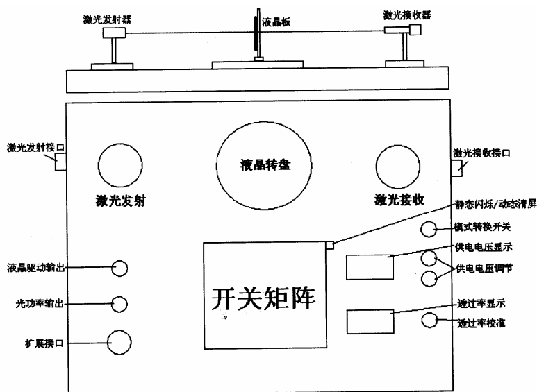
图 6 液晶光开关电光特性综合实验仪功能键示意图
