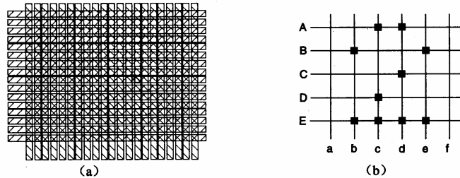
图 5. 液晶光开关组成的矩阵式图形显示器
