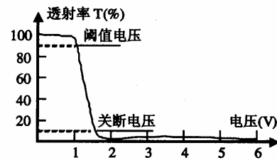
图 2 液晶光开关的电光特性曲线
